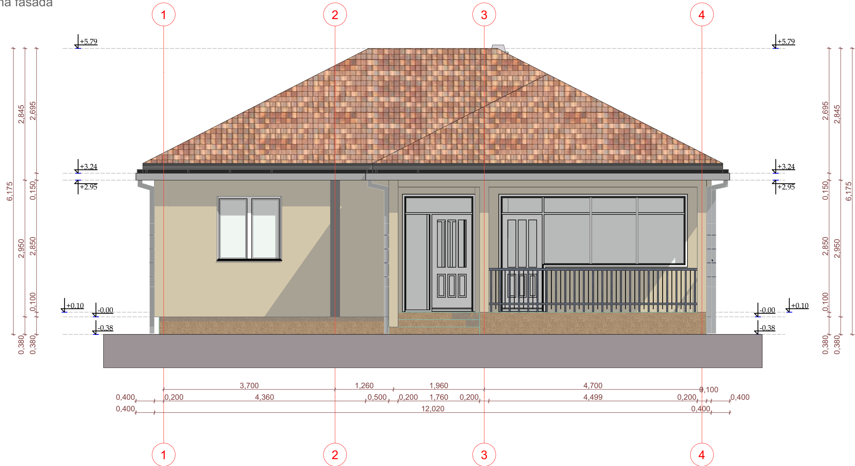
Zapadna fasada
