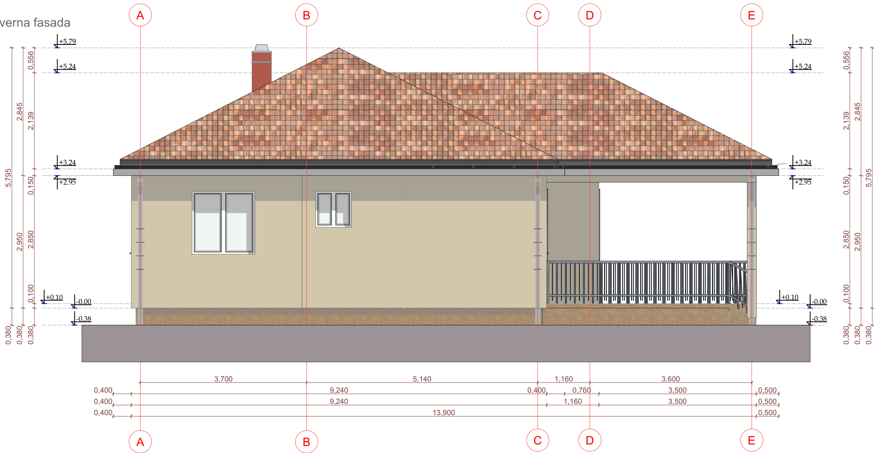
Južna fasada
