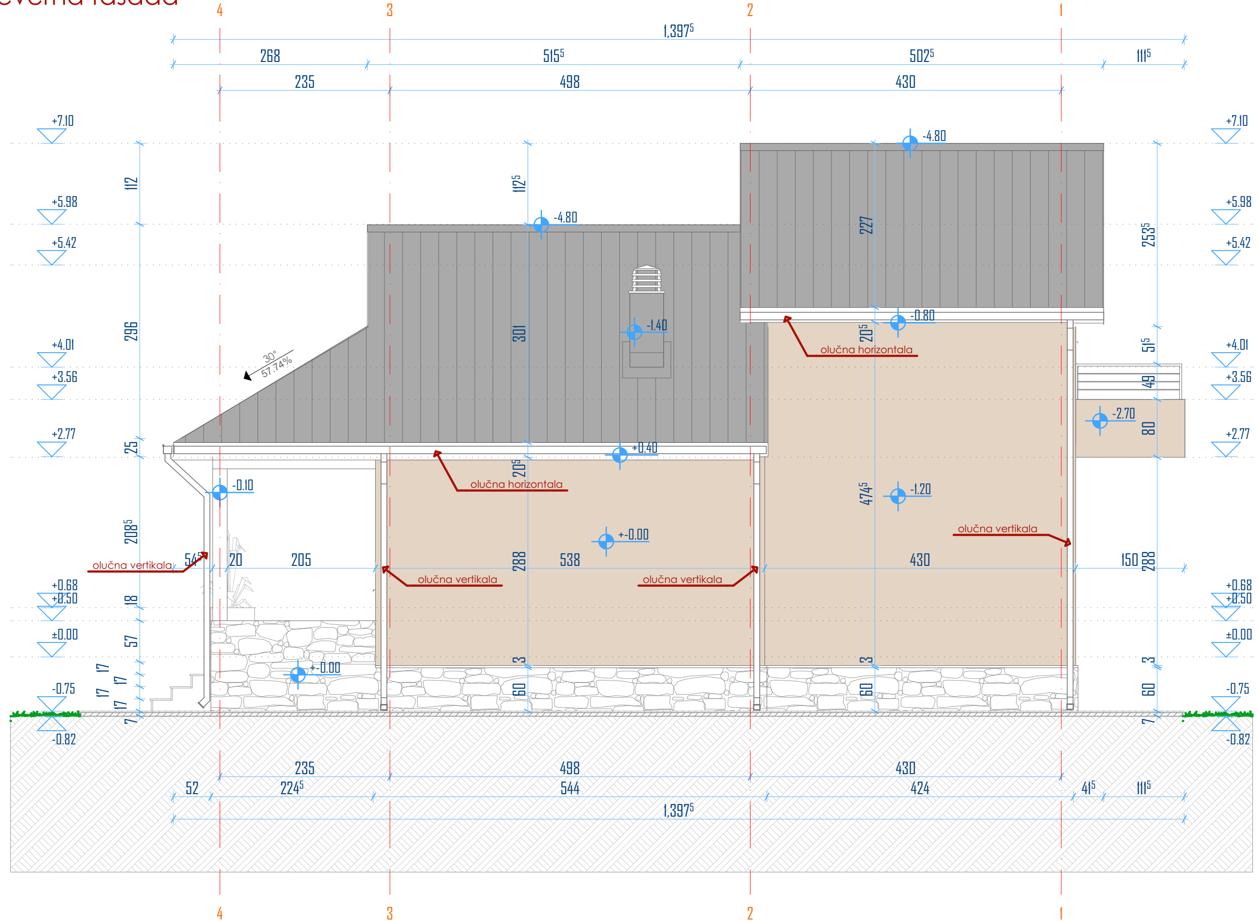
sjeverna fasada
