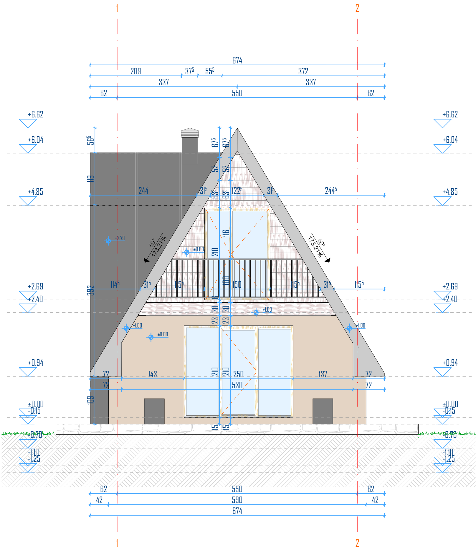
Južna fasada
