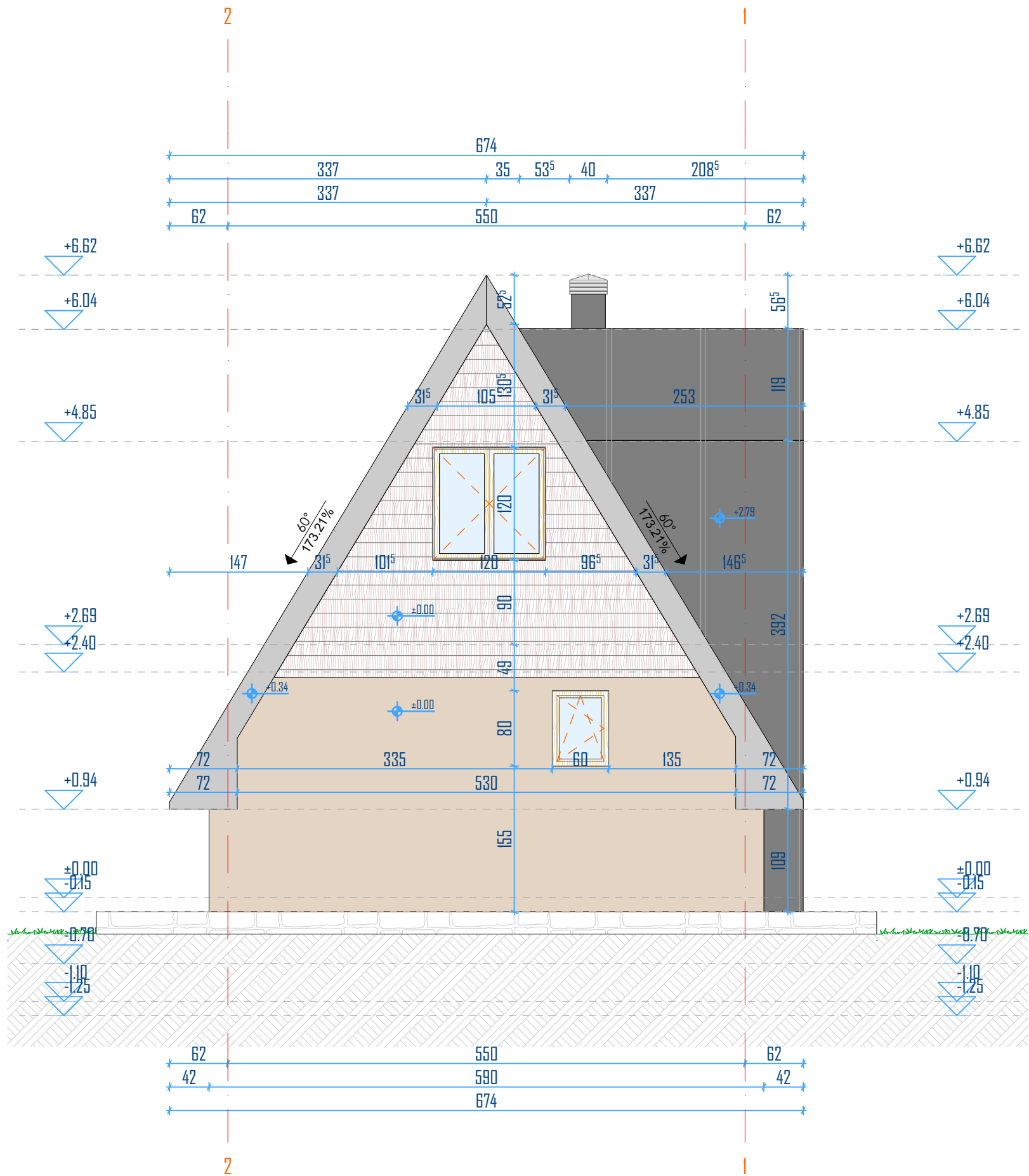
Sjeverna fasada
