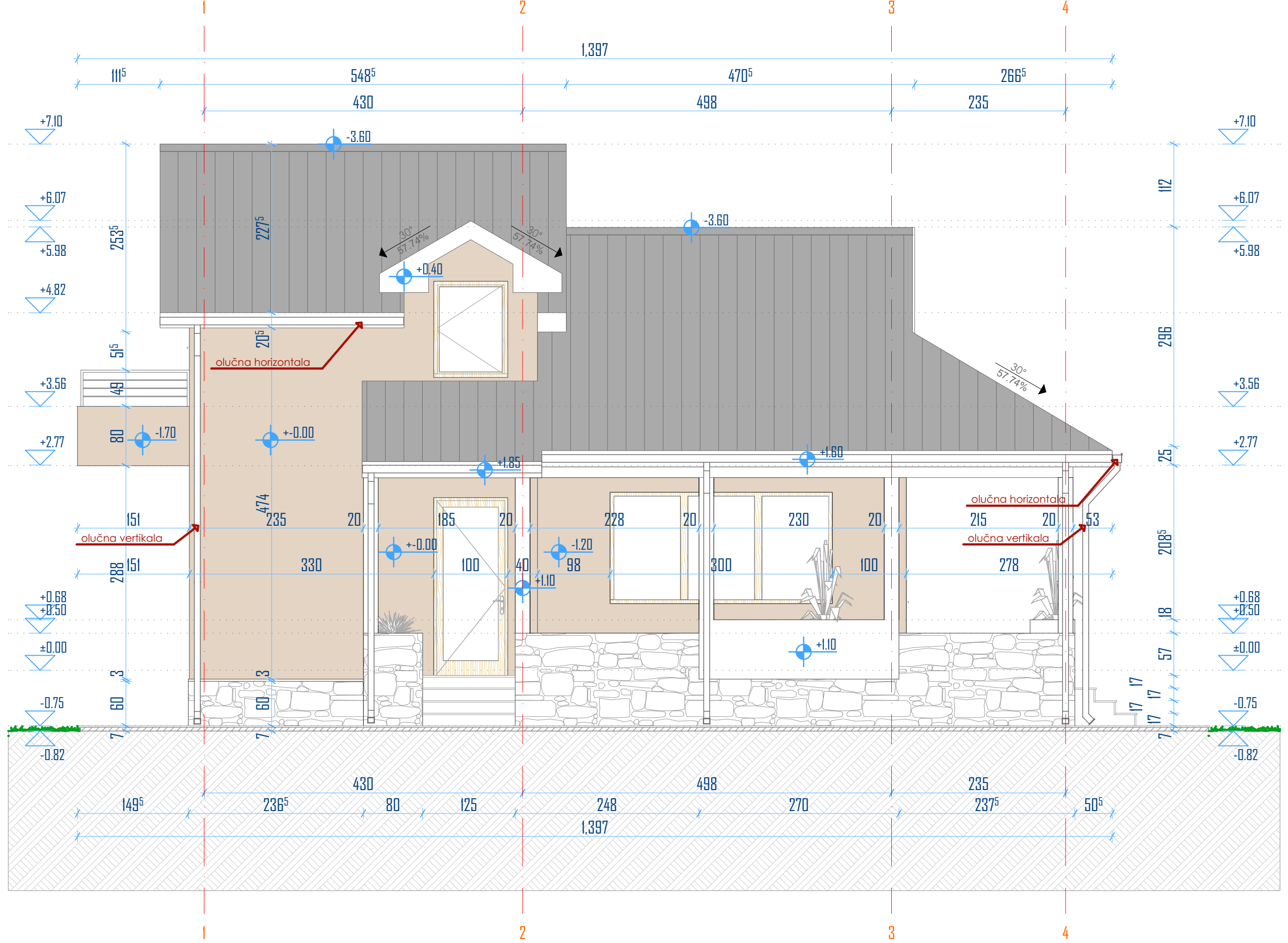
južna fasada
