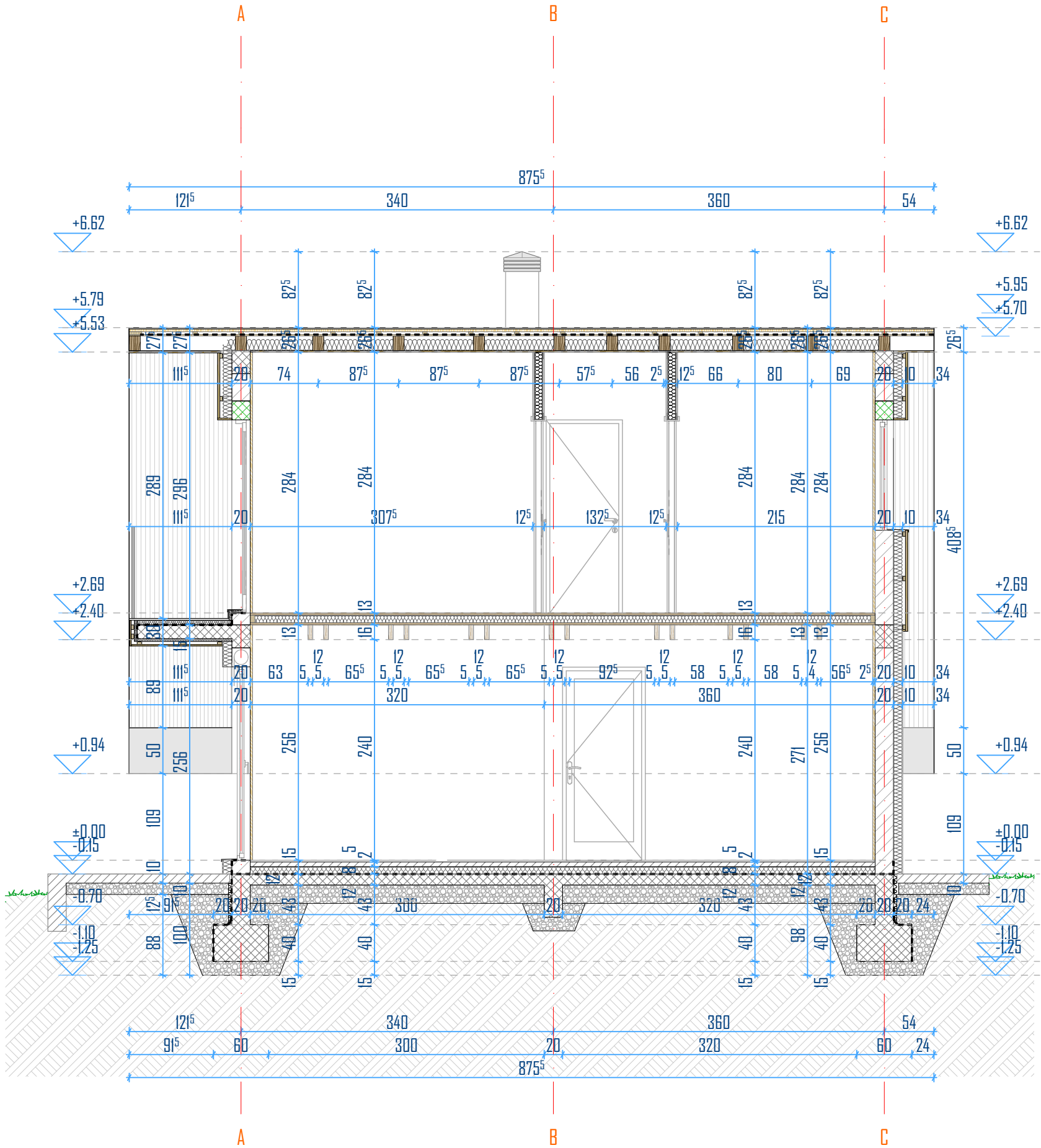
presjek 2-2
