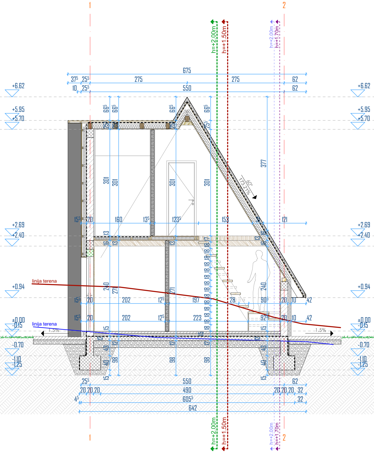
presjek 1-1
