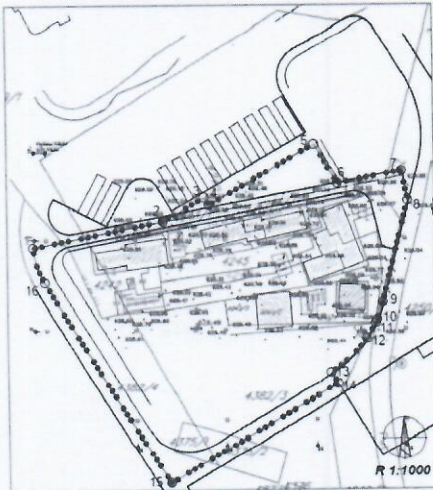
TOPOGRAFSKO KATASTARSKI PLAN
