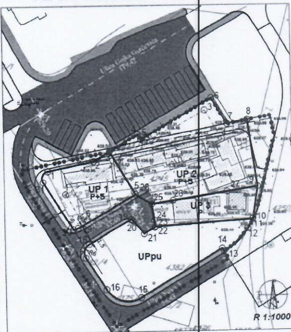
PLAN PARCELACIJE I REGULACIJE
