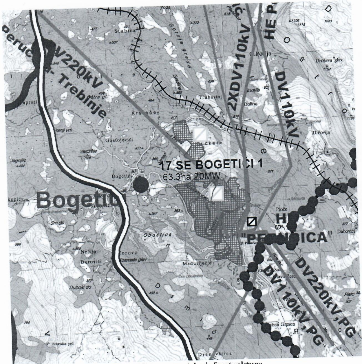
Plan elektroenergetske infrastrukture
