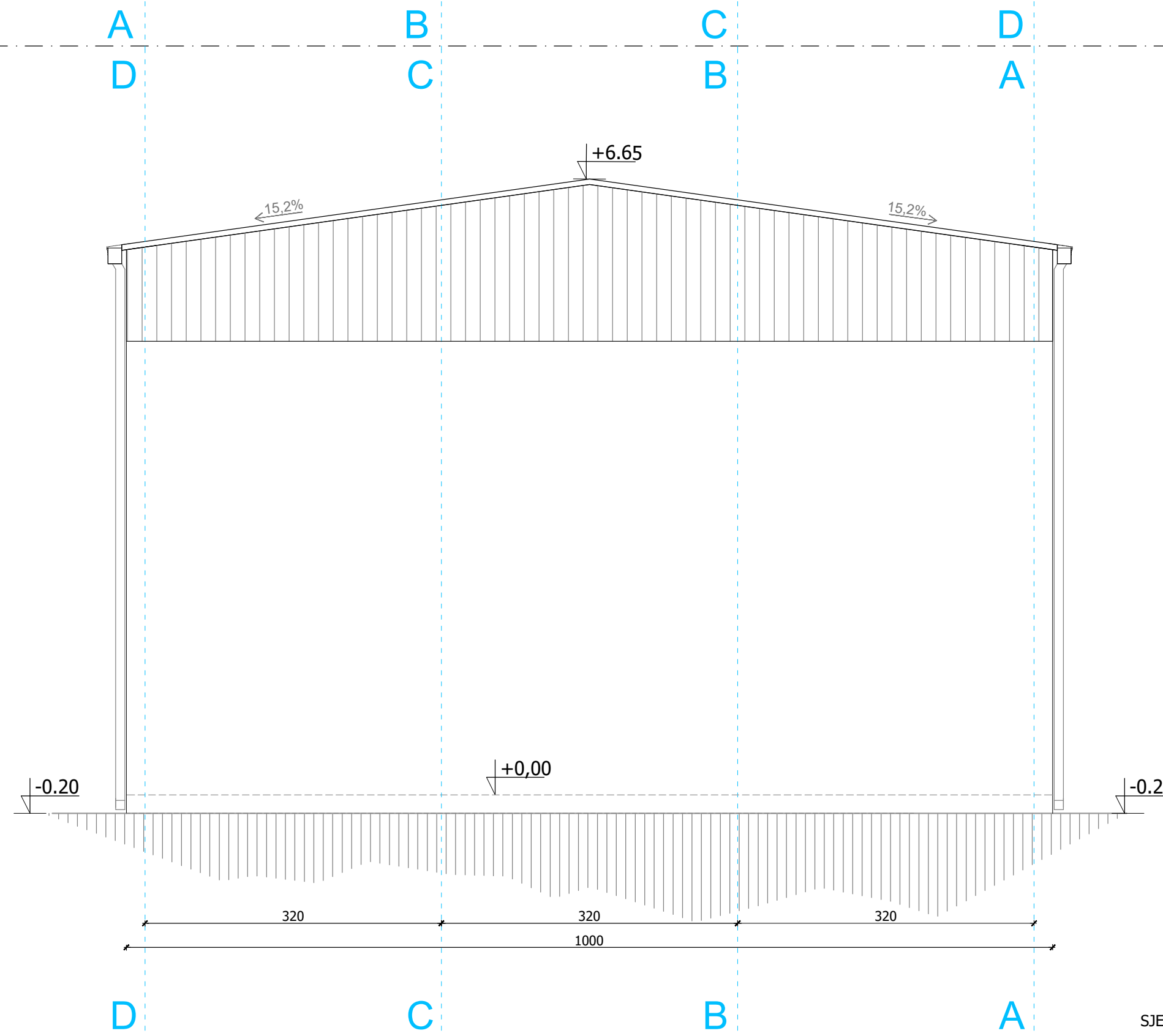
JUGOISTOČNA FASADA
