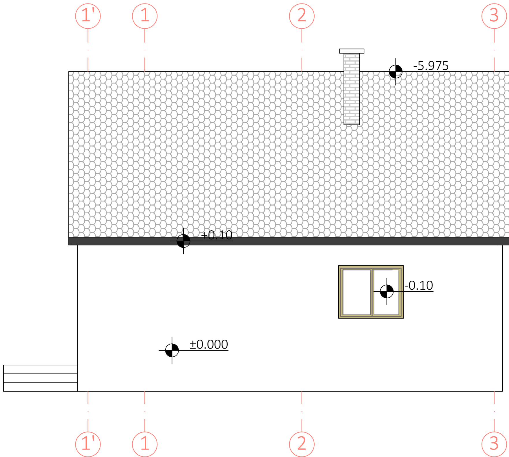
ISTOČNA FASADA
