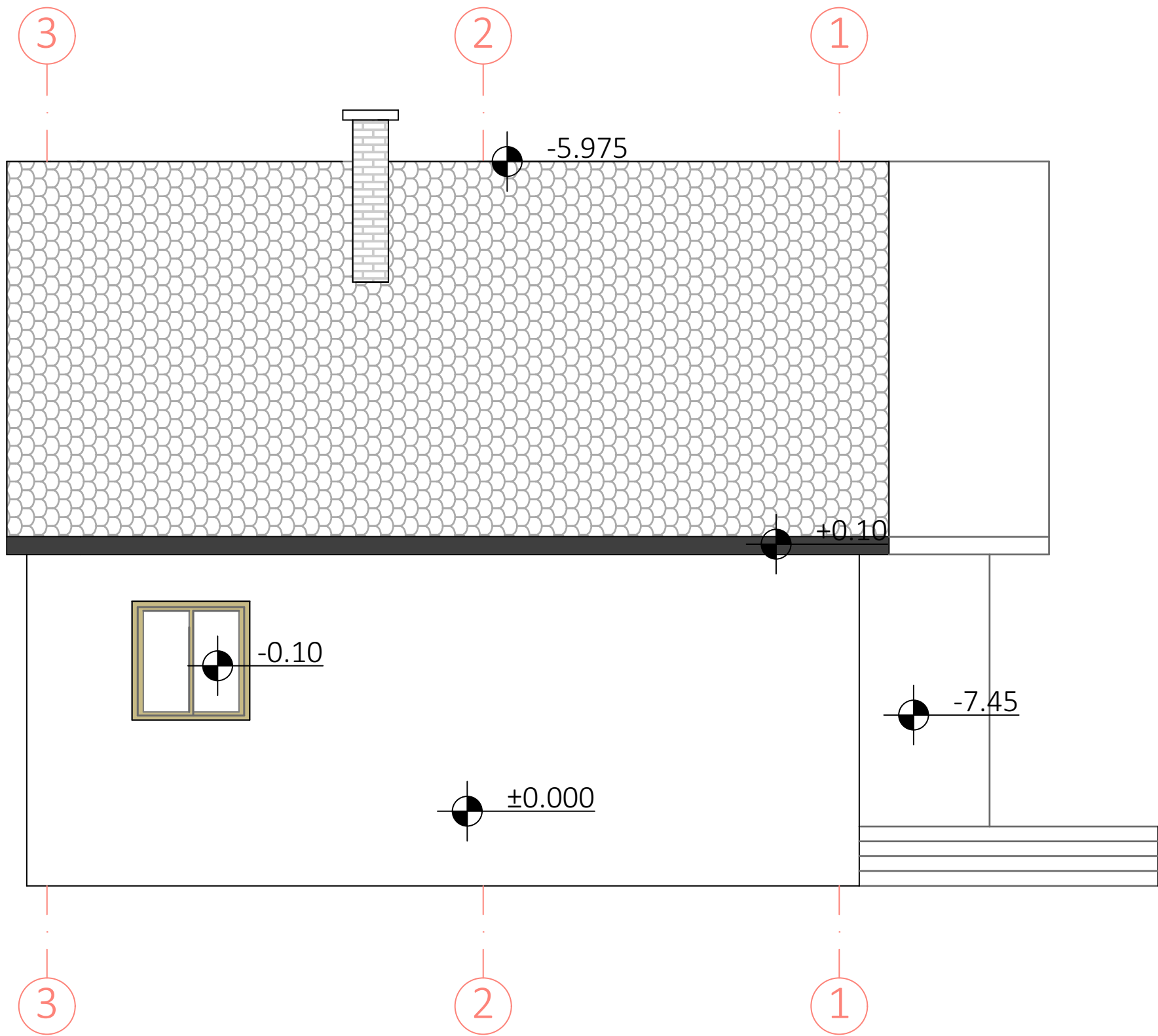
ZAPADNA FASADA
