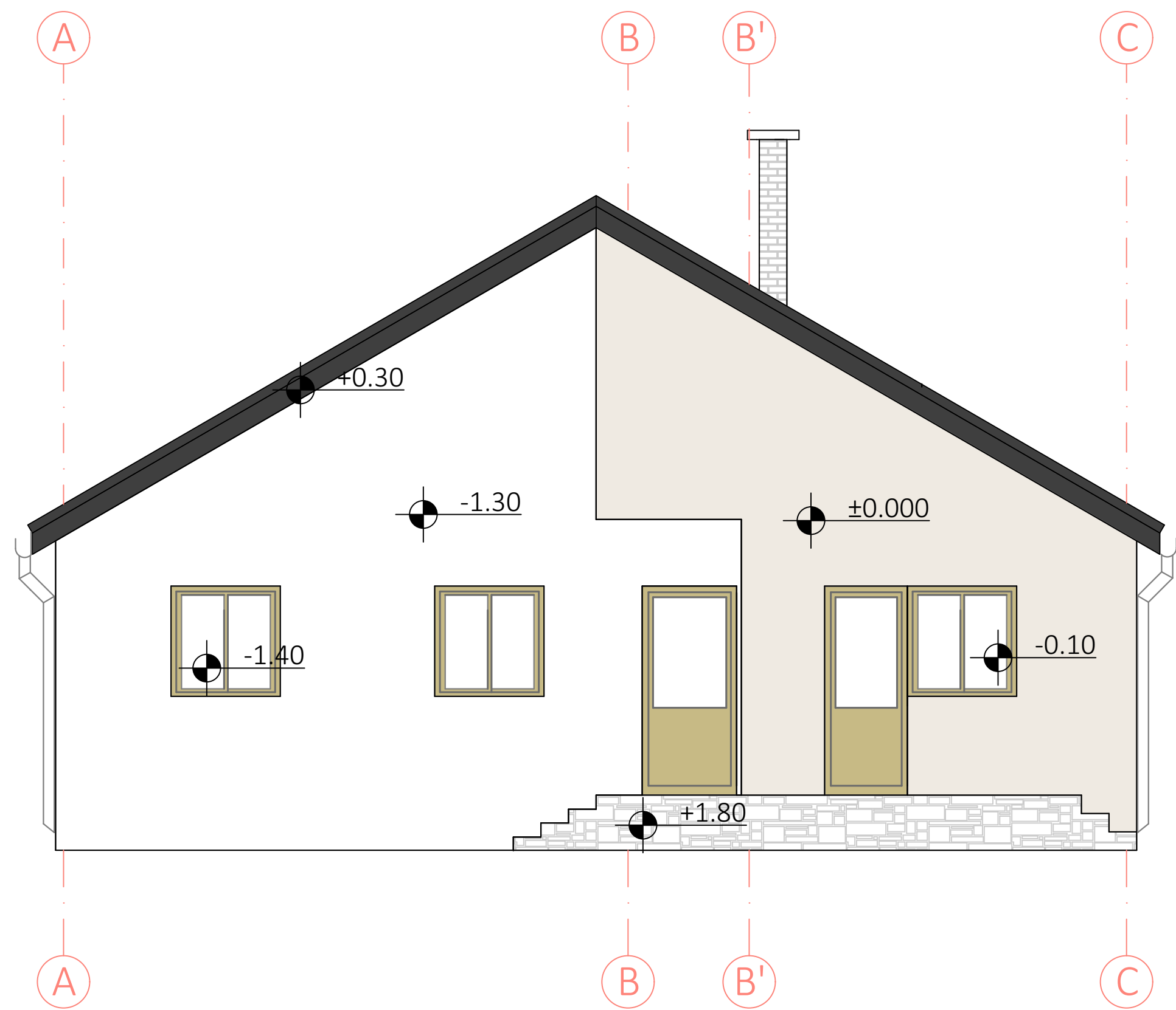
JUGOISTOČNA FASADA
