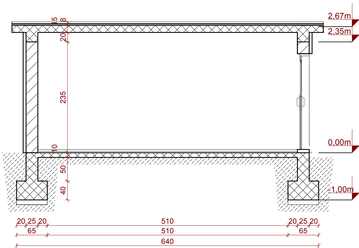
Presjek B-B
