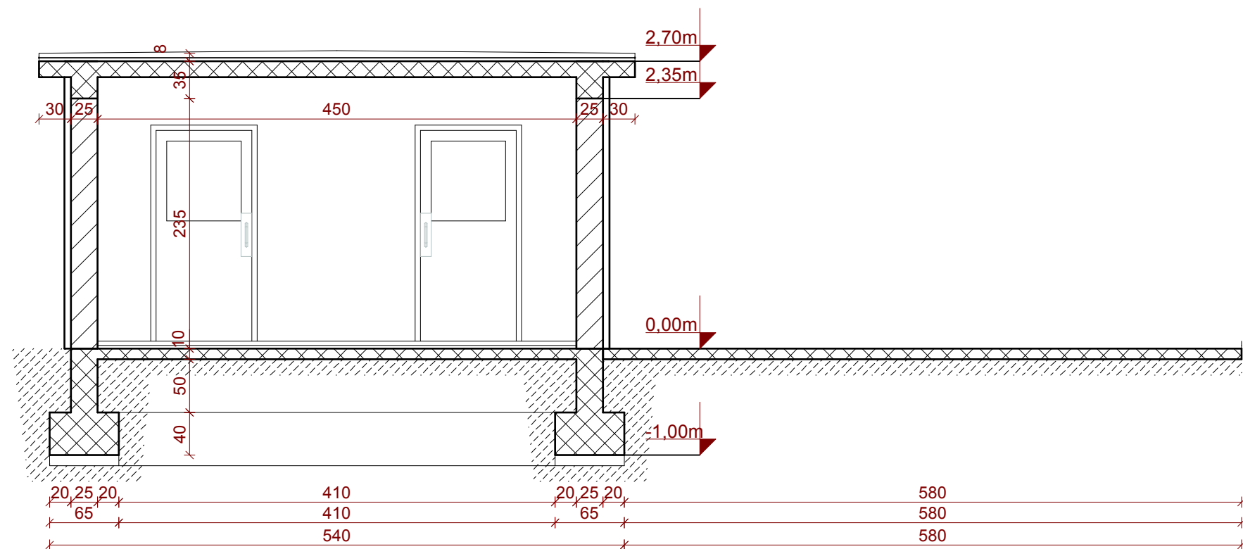
Presjek A-A
