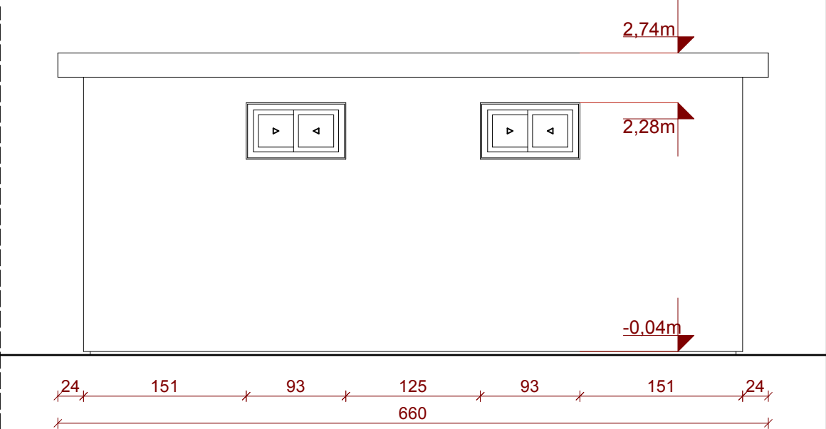
Presjek B-B
